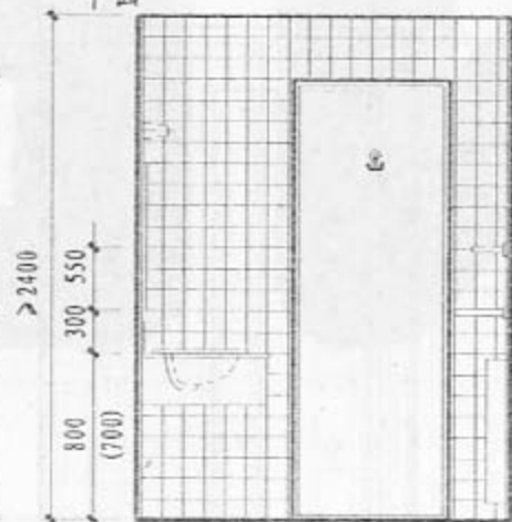
3-3剖面
