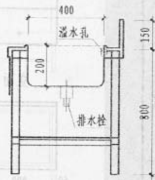
剖面
