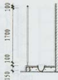
3-3 剖面
