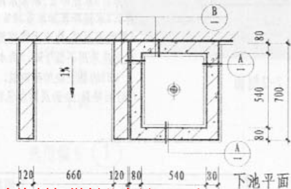
平面
