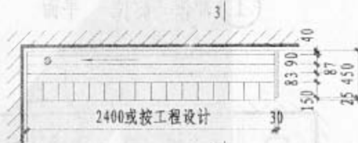
3-3剖面
