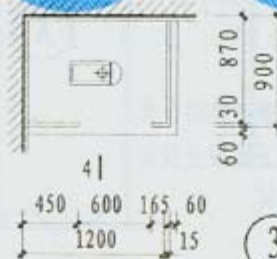
4-4剖面
