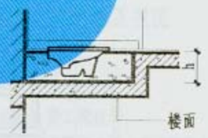
4-4剖面 (按连体型蹲便器绘制)
