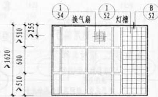
用于3型客房卫生间 ③ ⑧ ⑪ ⑫ ⑬ ⑭ ⑮ ⑯ ⑰ ⑱ ⑲ ⑳ ㉑ ㉒ ㉓ ㉔ ㉕ ㉖ ㉗ ㉘ ㉙ ㉚ ㉛ ㉜ ㉝ ㉞ ㉟ ㊱ ㊲ ㊳ ㊴ ㊵ ㊶ ㊷ ㊸ ㊹ ㊺ ㊻ ㊼ ㊽ ㊾ ㊿
