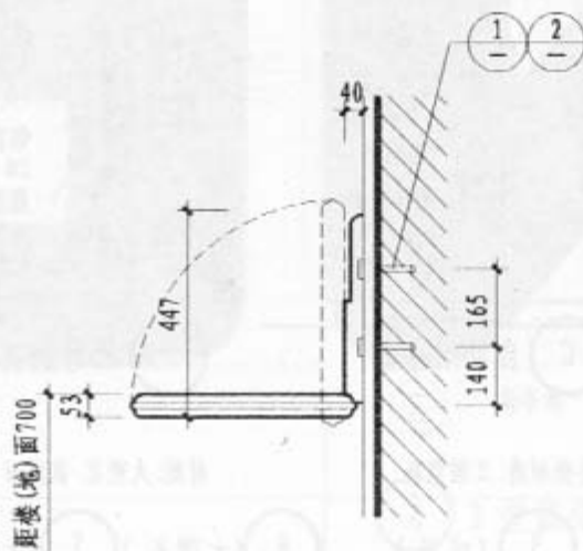
剖面
