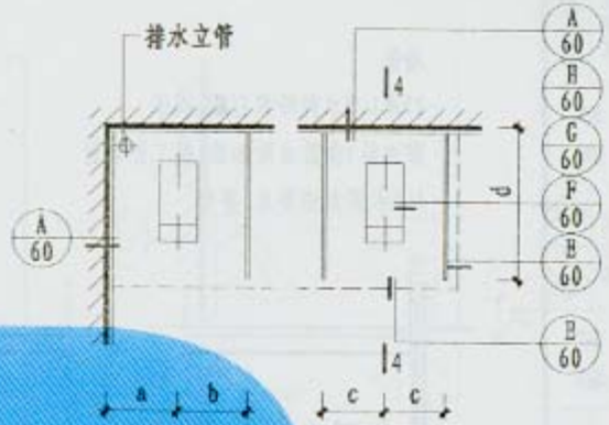
平面 ⑤
