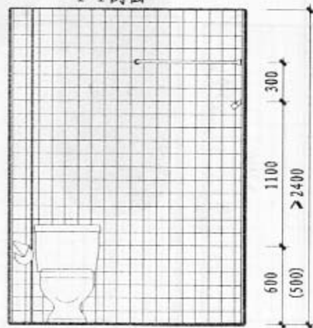
4-4剖面
