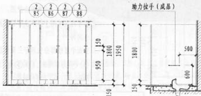
2-2 剖面
