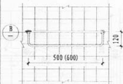
立面
