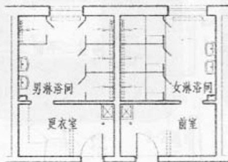
2型淋浴间
