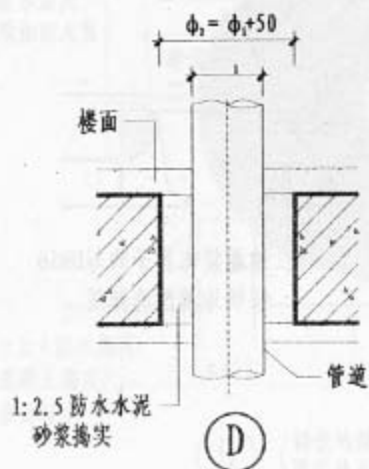
管道穿楼板
