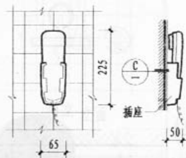
立面
