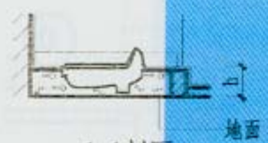
1-1剖面 (按普通型蹲便器绘制 亦适用于幼儿型蹲便器)
