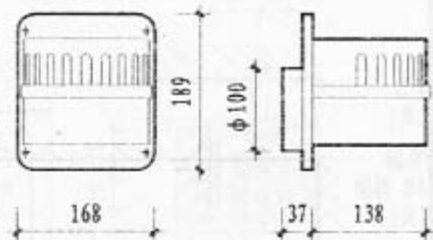
换气扇(成品)
