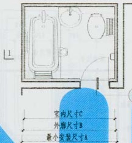
平面 (BU1620型)
