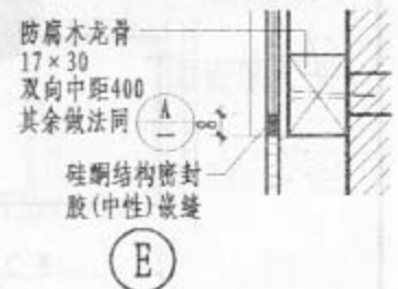
梳妆镜详图(四)
