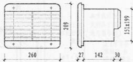
换气扇(成品)
