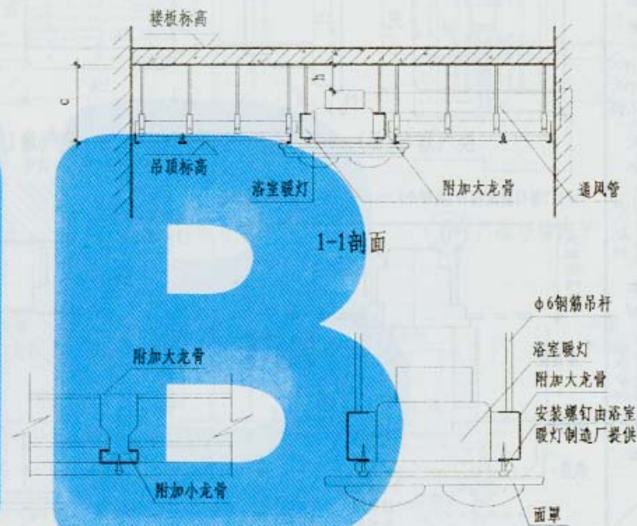
1 附加大、小龙骨连接方式 2 浴室暖灯与附加大龙骨连接方式
