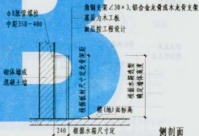
① 隐蔽式水箱洁具的建筑装修详图
