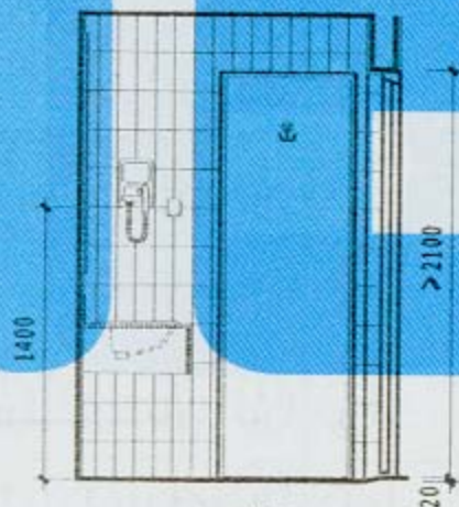
5-5剖面
