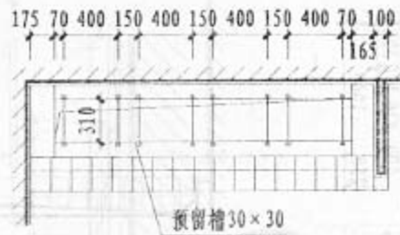
幼儿坐厕平面 (混凝土沟壁预留槽位置)
