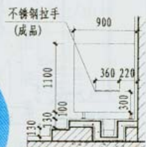
2-2剖面(用于地面)
