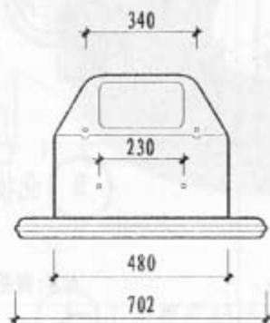
立面
