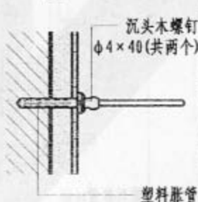
平面
