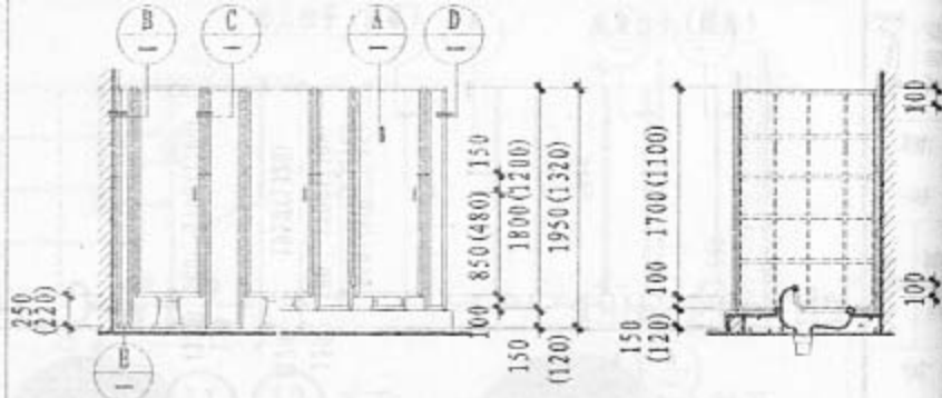
立面(落地式隔断)
