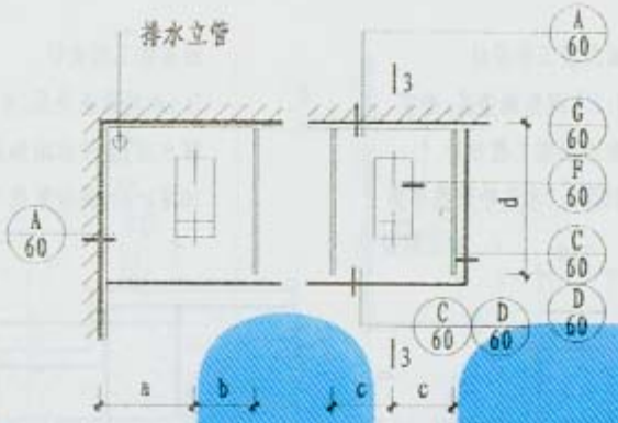
平面 ④
