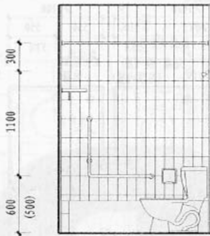
3-3 剖面
