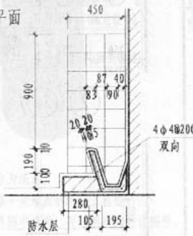
3-3剖面
