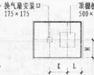
顶棚板开口位置图
