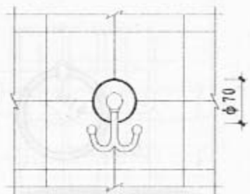
立面
