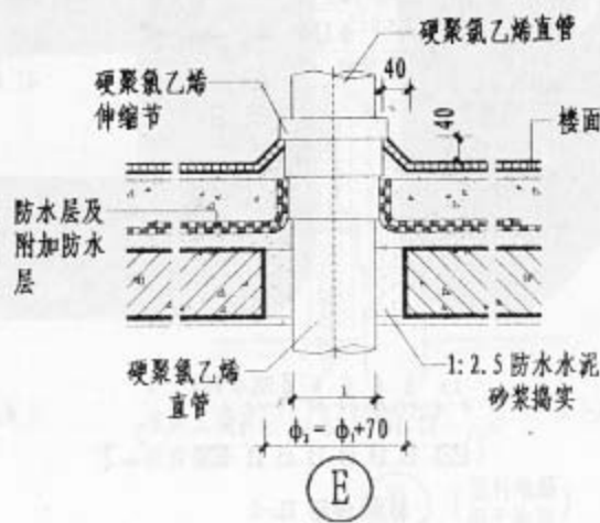
硬聚氯乙烯伸缩节穿防水楼板
