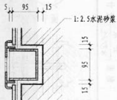
④ 纸巾盒
