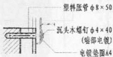
塑料胀管 φ8x50 (四个)
