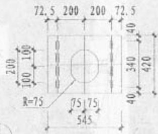
幼儿坐厕平面 (混凝土沟壁预留槽位置)
