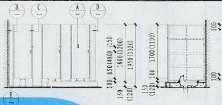
2 立面(落地式隔断)
