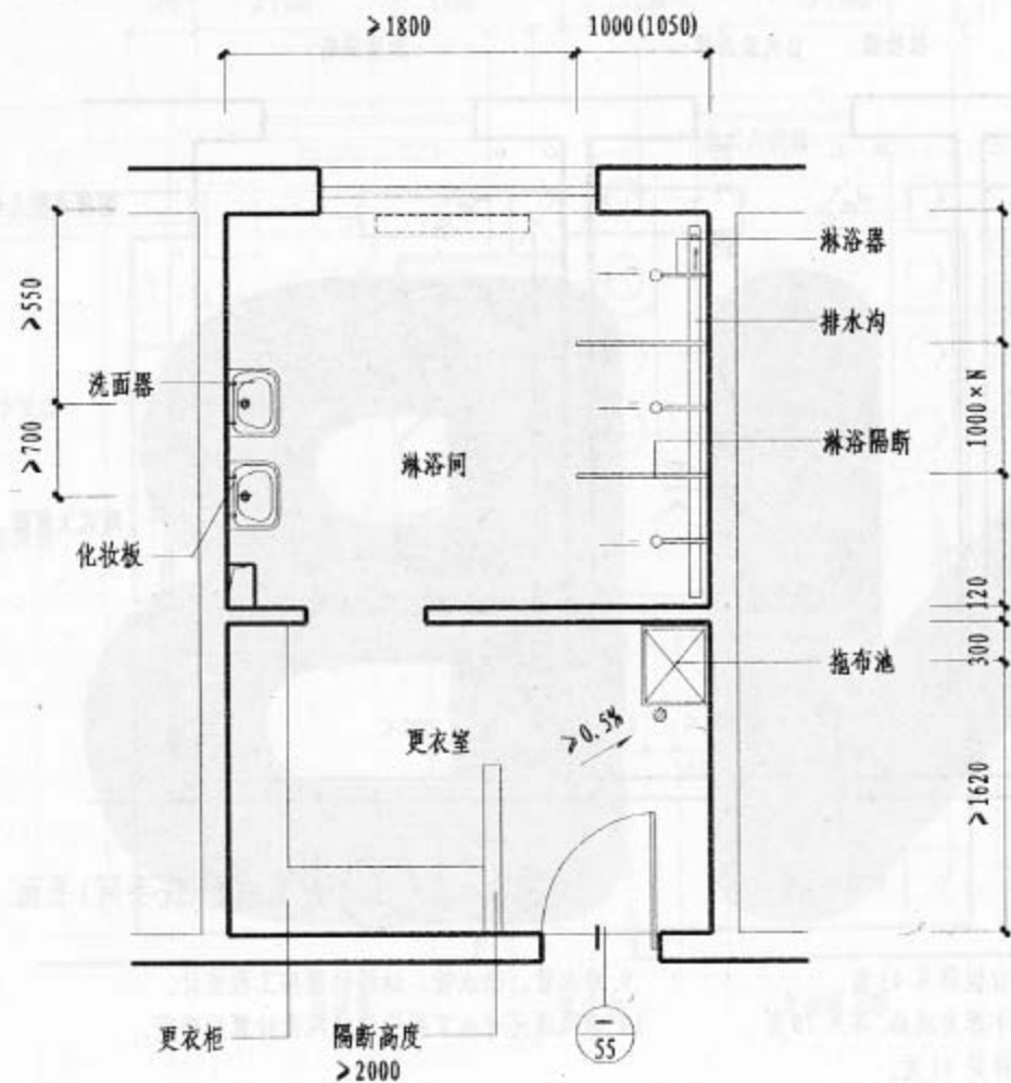
1 型淋浴间平面
