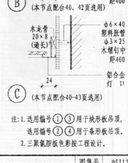
客房卫生间灯槽详图
