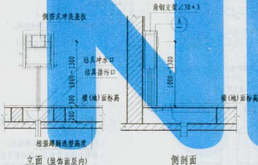
③ 隐蔽式水箱洁具安装(前按式,配蹲厕)
