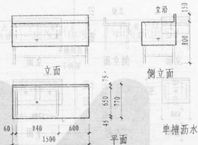
③ (有立沿)
