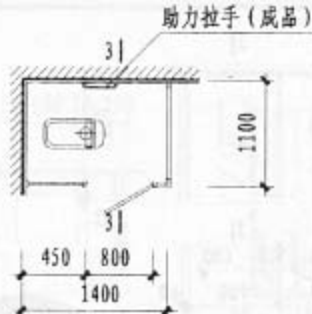
10 11 12 平面
