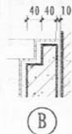
木格栅大样
