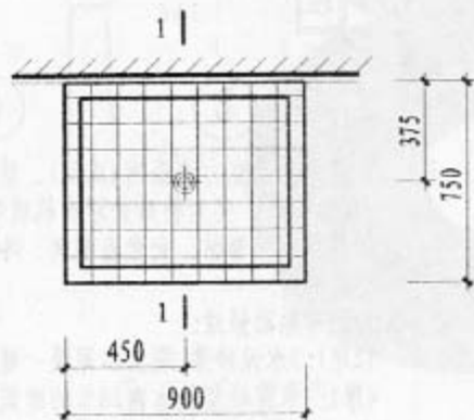
平面
